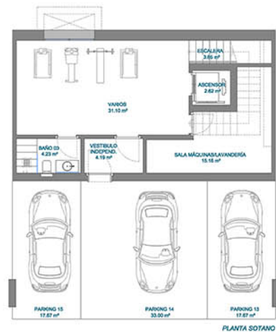
PLANTA SOTANO
